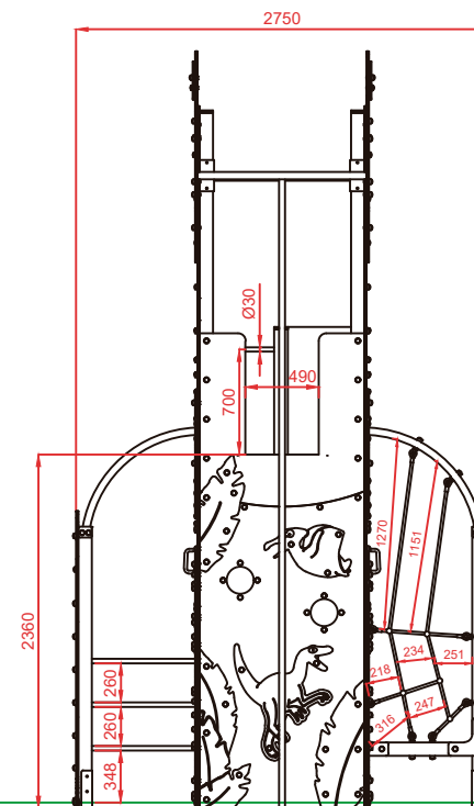
PERFIL
