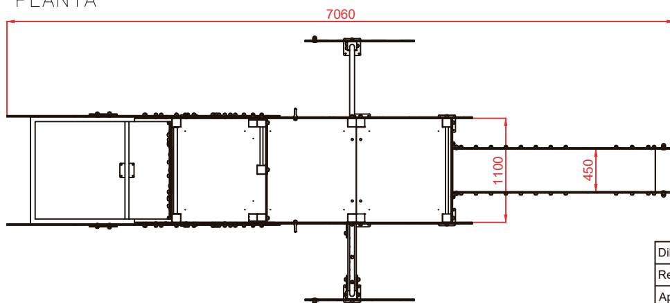
PLANTA
