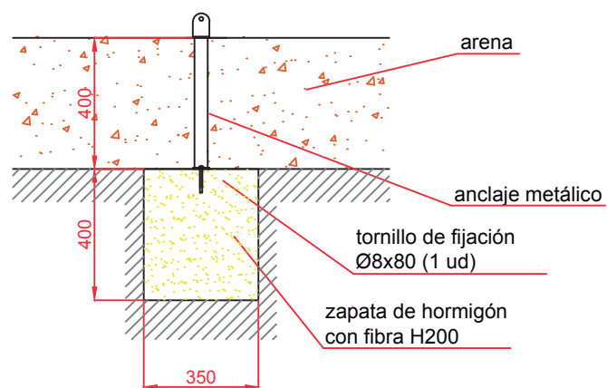
ESQUEMA DE CIMENTACIÓN EN HORMIGÓN E: 2/1
