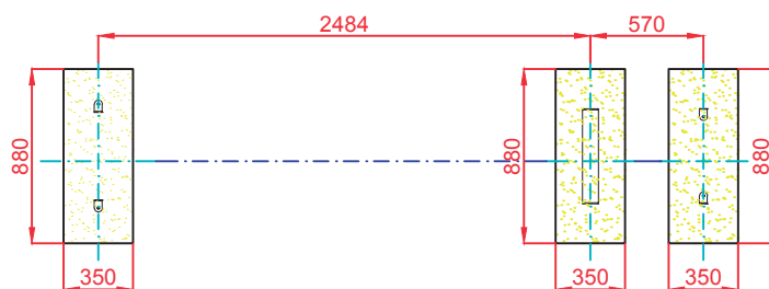
PLANTA CIMENTACIÓN
