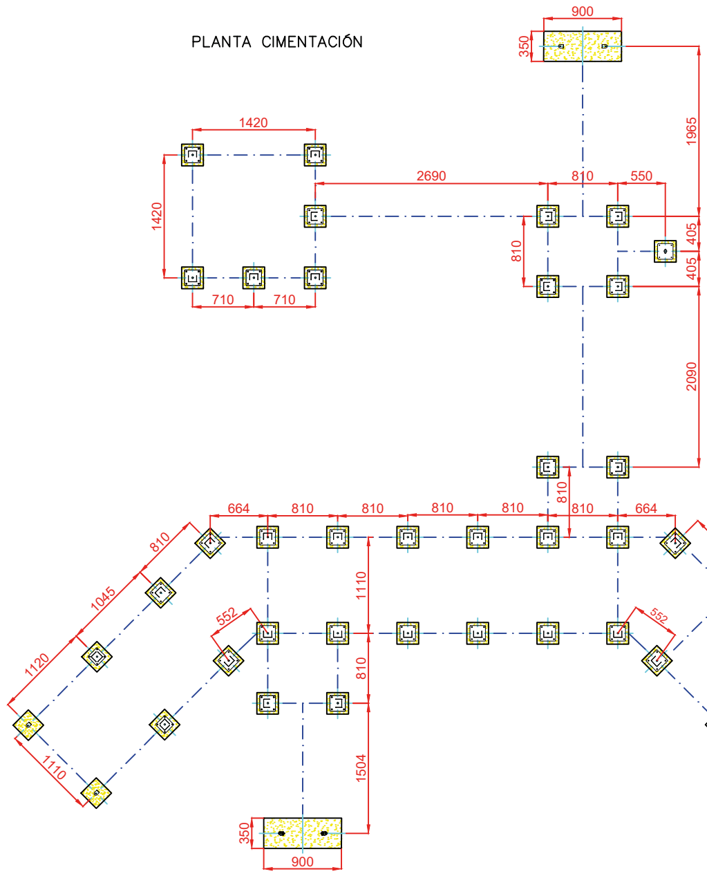
ESQUEMA DE CIMENTACIÓN EN ARENA E: 2/1
