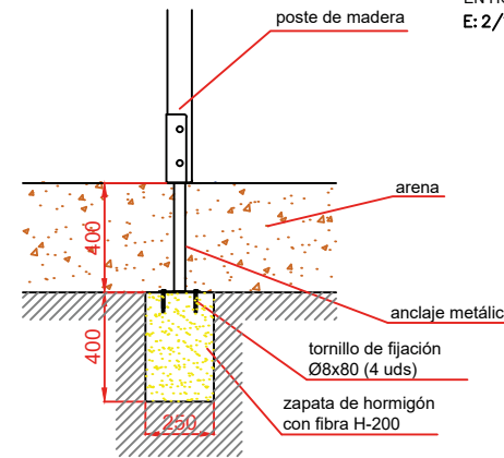
ESQUEMA DE CIMENTACIÓN EN ARENA E: 2/1
