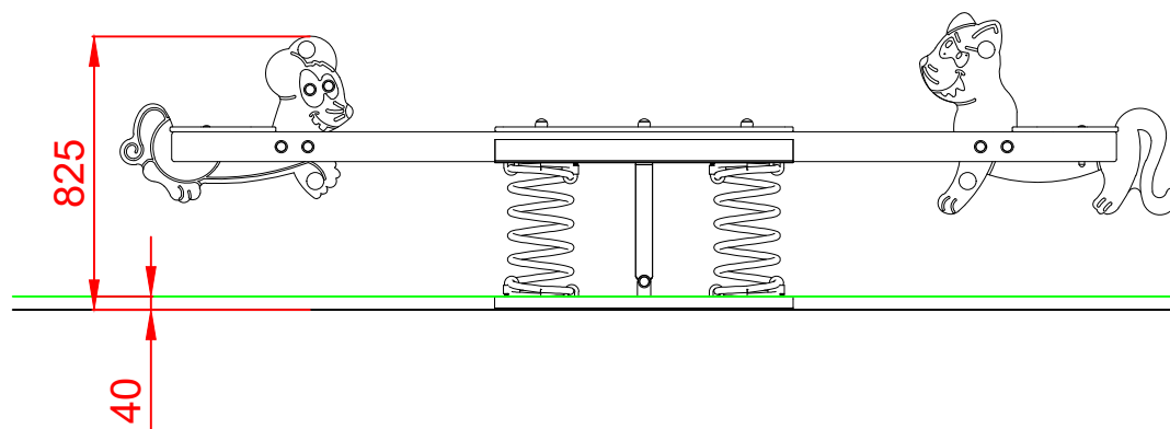
ALZADO
