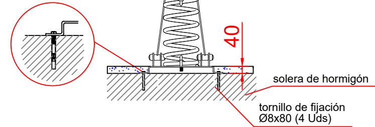
Detalle de sujeción de espirro metálico
