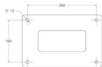
detalle anclaje 1.5
