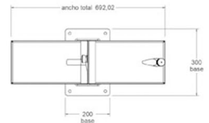
detalle anclaje 1.5
