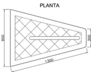
ISLETA CON PANEL DIRECCIONAL MEDIDAS: 1300x950x900 mm
