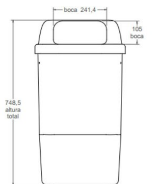
vista alzado 1:10
