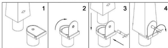
SECUENCIA ENCASTRE BOLARDO
