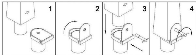
SECUENCIA ENCASTRE BOLARDO
